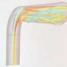
90° Bogen über konditioniertes Profil
